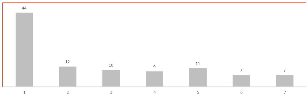
VRAAG 3- Levels 1-7
