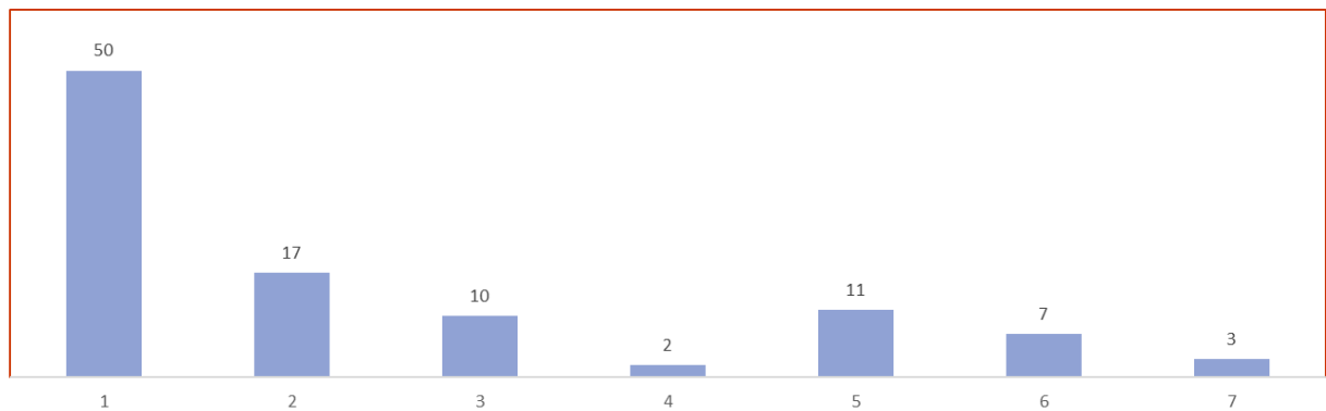
VRAAG 2- Levels 1-7
