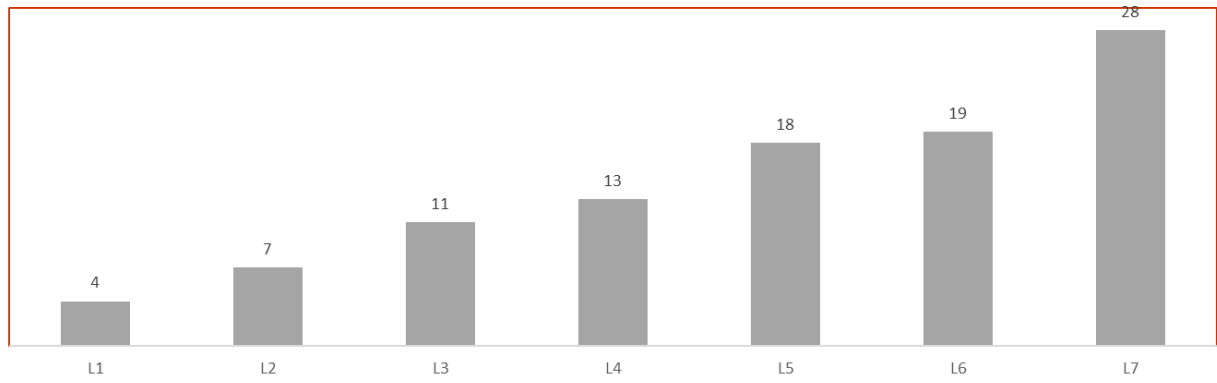
VRAAG 1- Levels 1-7
